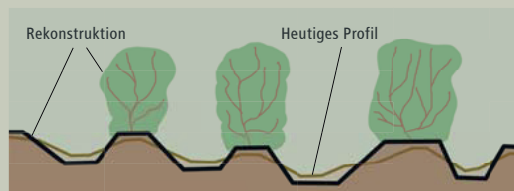
Querschnittsprofil der Landwehr. Aufnahme: Dipl.-Ing. Hans-Joachim Pinnow, öffentlich bestellter Vermessungsingenieur Radevormwald 2013
